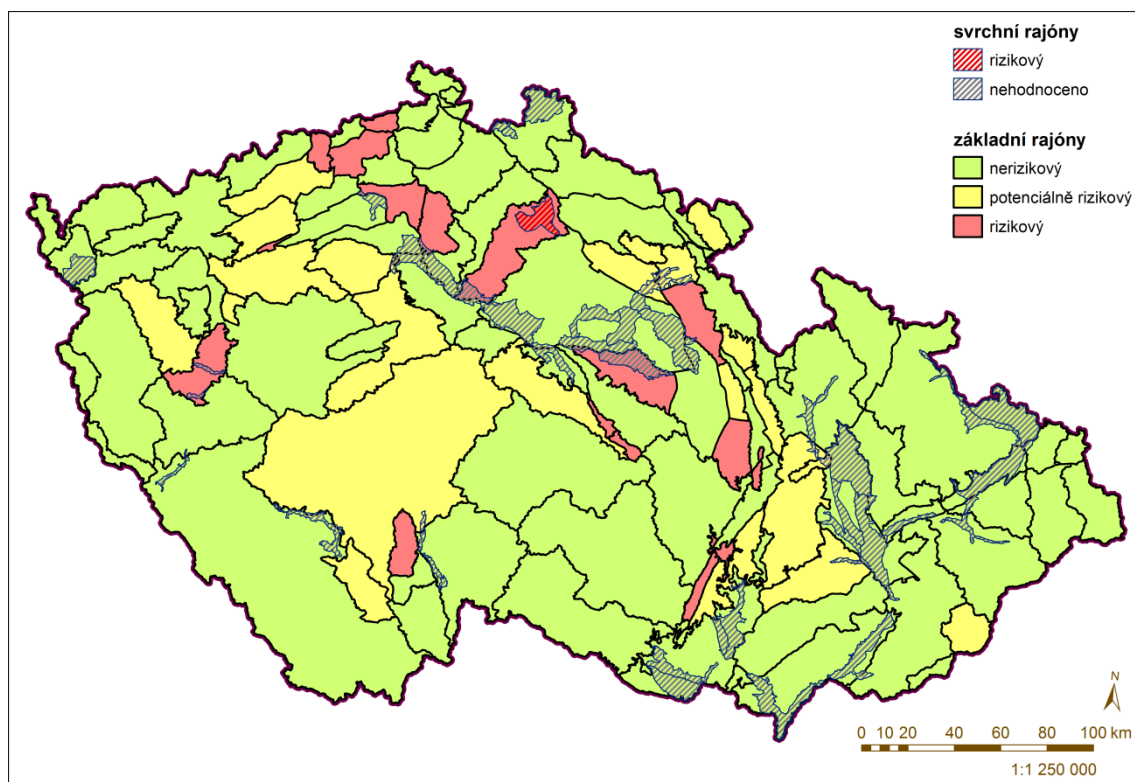
Obr. 8 Hydrogeologické rajony potenciálně zranitelné vůči nedostatku vody, zdroj: VÚV
