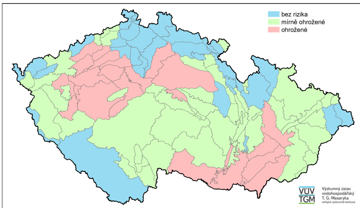
Obr. 6 Regionalizace zranitelnosti hydrogeologických rajonů vůči suchu stanovená podle velikosti průměrného základního odtoku za období 1981–2010, zdroj: VÚV
