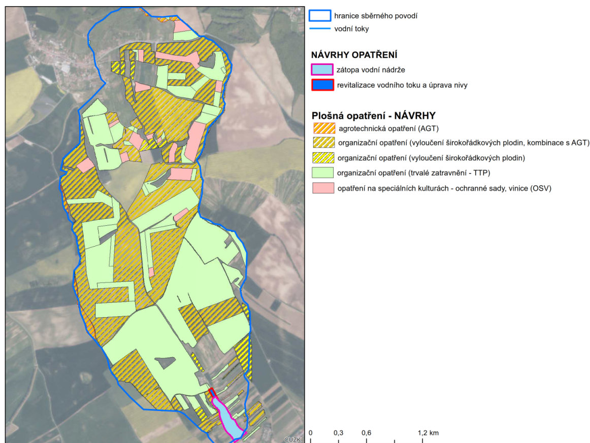
Obrázek 3: Navržená společná zařízení na ortofoto (Zdroj: ČÚZK)
