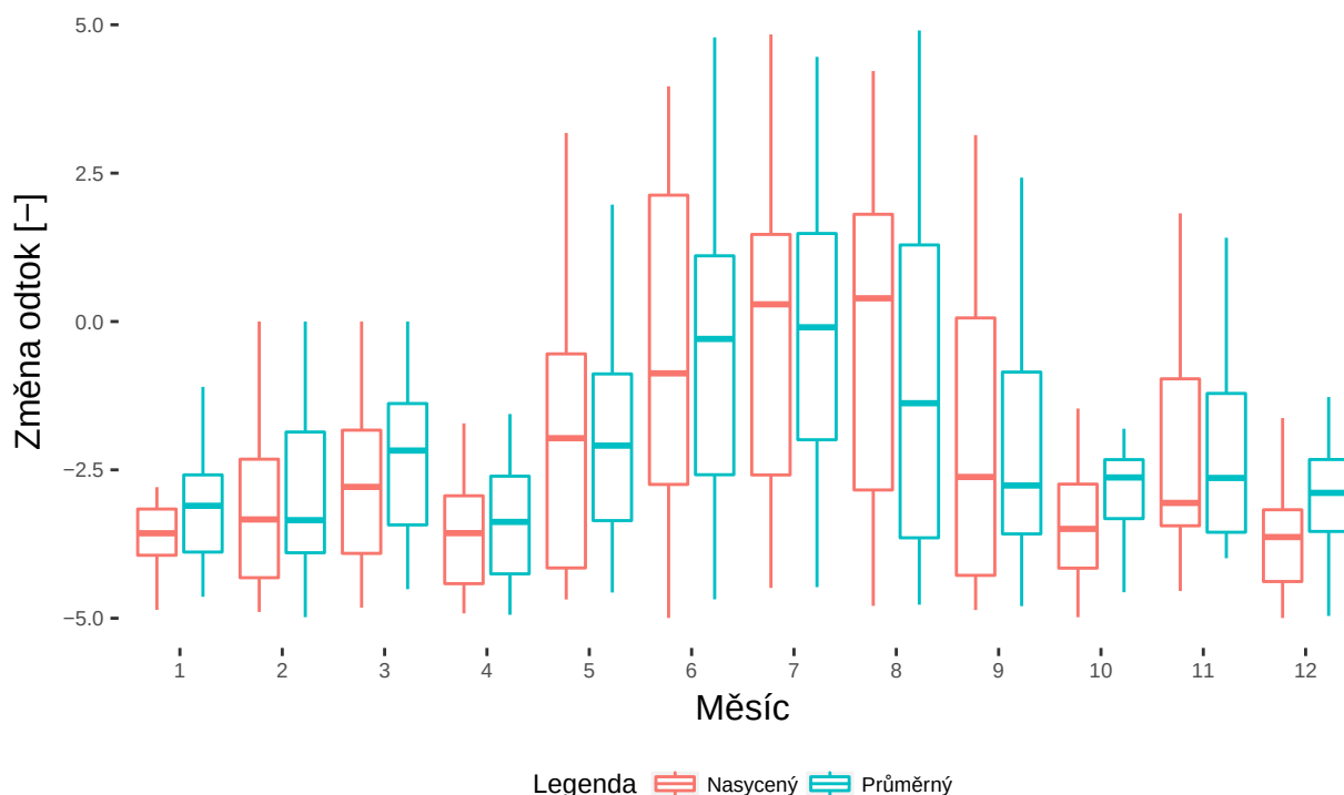
Obrázek 13: Změny měsíčních odtokových výšek ve formě boxplotů (pře opatřeními a po realizaci opatření)
