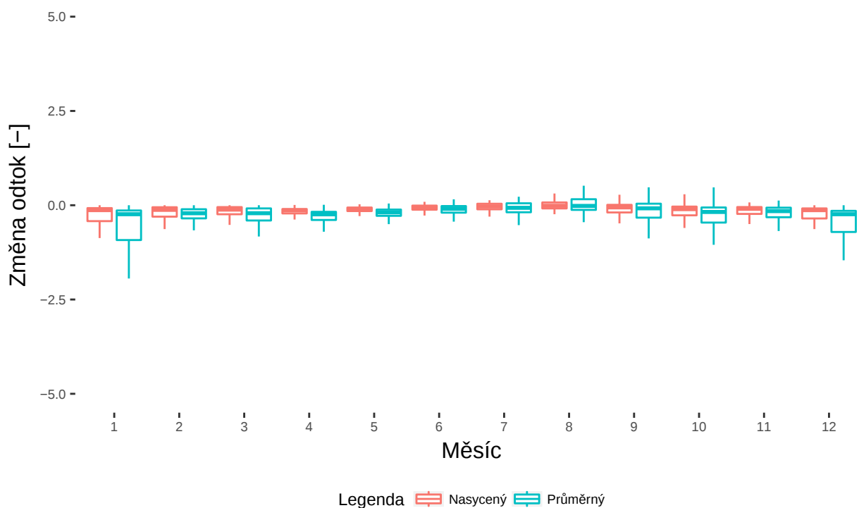
Obrázek 14: Změny měsíčních odtokových výšek ve formě boxplotů (pře opatřením a po realizaci opatření)
