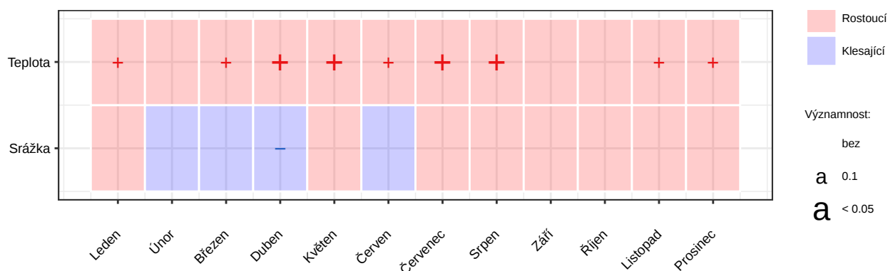
Obrázek 11: Analýza trendů srážek a teplot vzduchu pomocí Mann-Kendall testu
