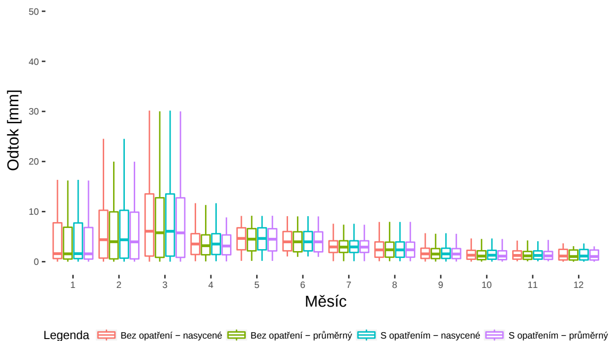
Obrázek 13: Průměrné měsíční odtokové výšky ve formě boxplotů pro jednotlivé varianty hodnocení
