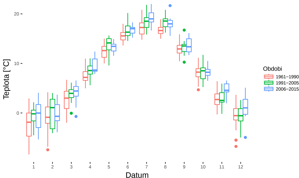
Obrázek 7: Průměrné měsíční teploty vzduchu za období 1961-1990, 1991-2005 a 2006-2015 ve formě boxplotů
