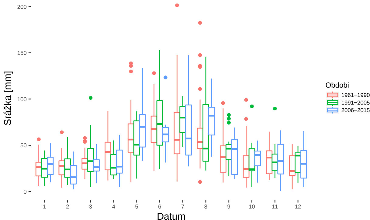
Obrázek 6: Měsíční srážkové úhrny za období 1961-1990, 1991-2005 a 2006-2015 ve formě boxplotů
