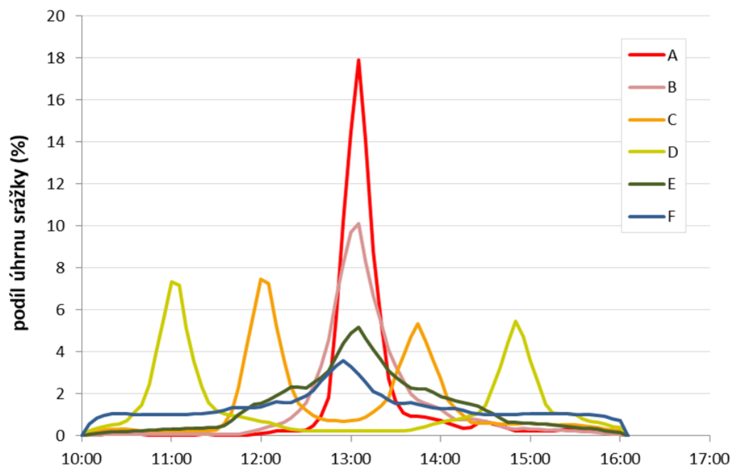
Obrázek 9: Průběh 5-min intenzit návrhových srážek
