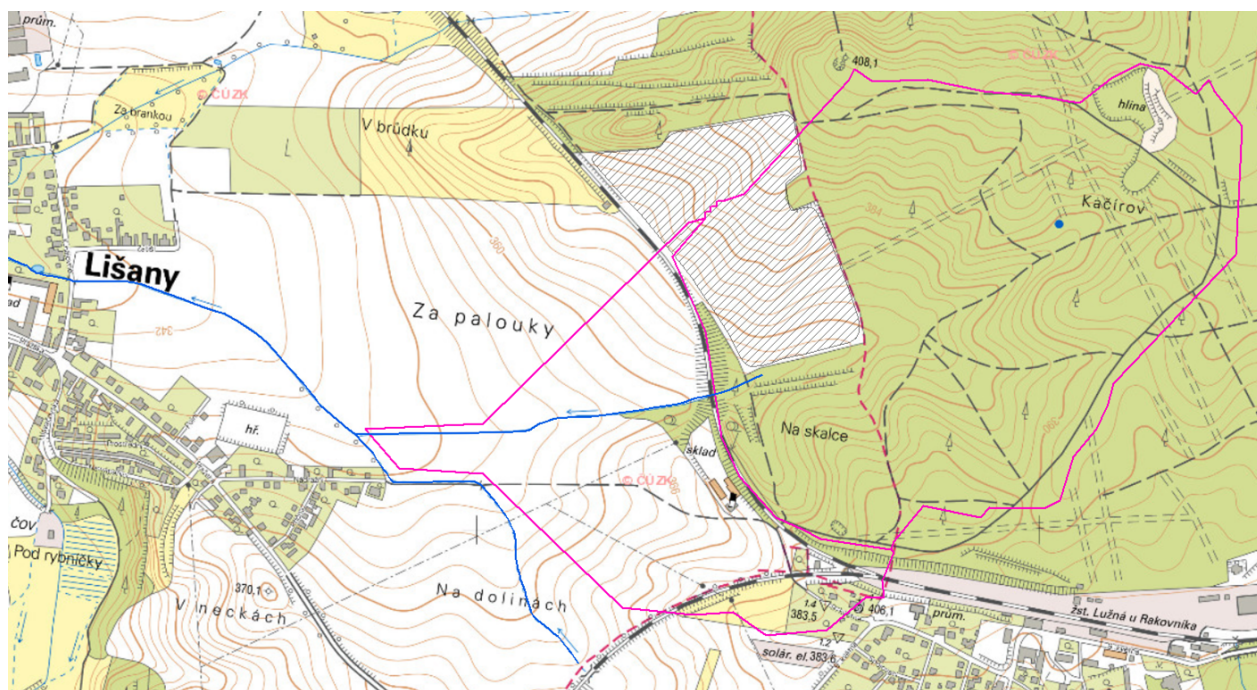
Obrázek 5: Lokalizace navrženého protierozního opatření ve střední části povodí bezejmenného levostranného přítoku Lišanského potoka ve formě agrotechnického opatření
