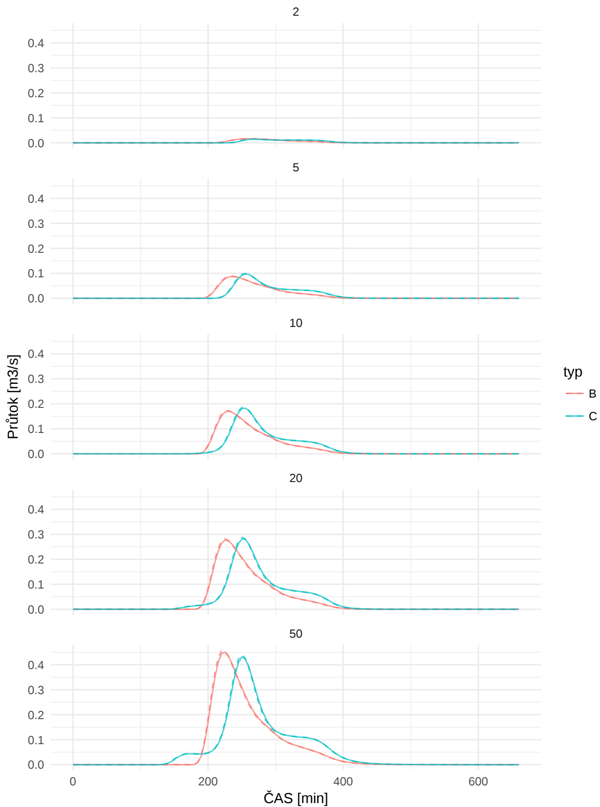
Obrázek 16: Návrhové průtoky dle N - letostí pro jednotlivé typy vln (čárkovaně-před opatřením, plně-po opatření)
