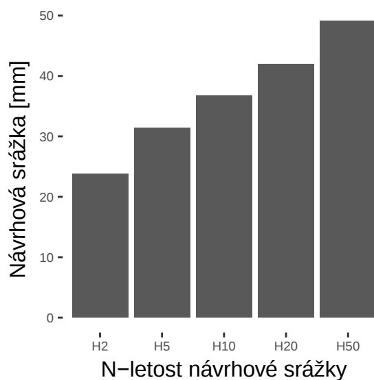
Obrázek 8: Návrhové srážky s dobou opakování 2, 5, 10, 20 a 50 let
