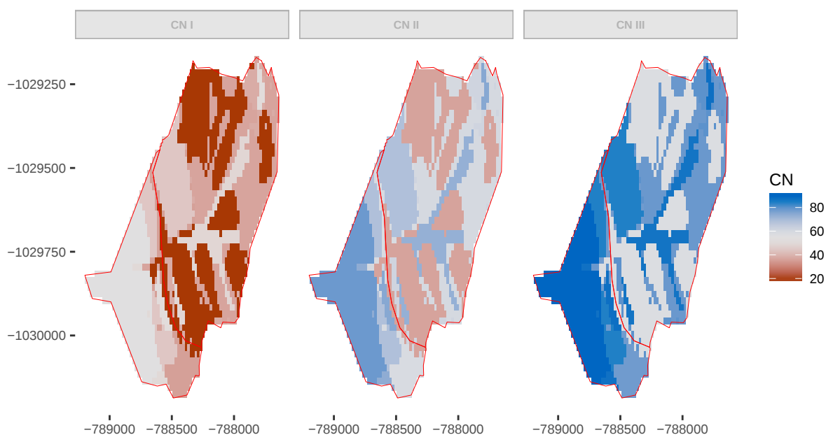
Obrázek 12: Hodnoty CN pro zájmové území a různé vláhové podmínky
