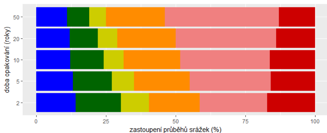
Obrázek 10: Rozdělení jednotlivých typů návrhové srážky
