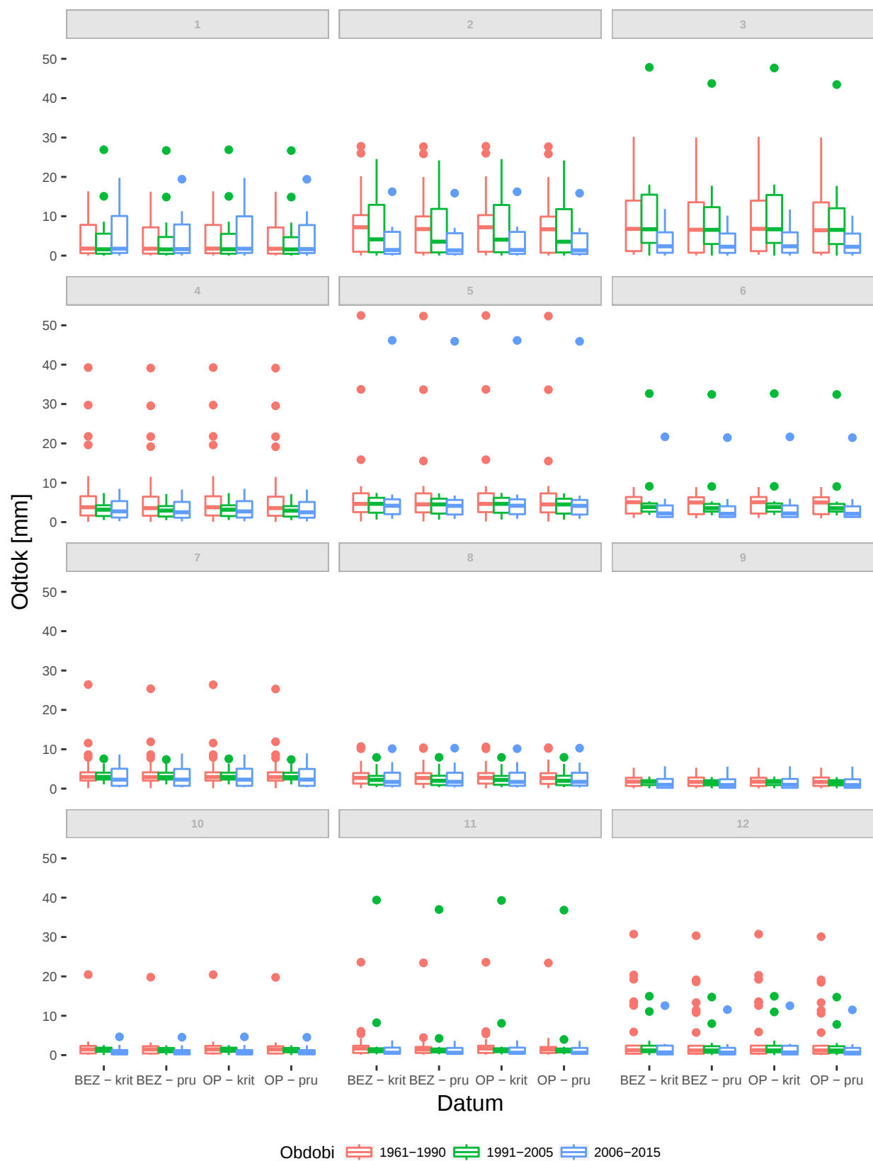
Obrázek 15: Měsíční odtokové výšky za období 1961-1990, 1991-2005 a 2006-2015 ve formě boxplotů bez opatření (BEZ) a s opatřením (OP)
