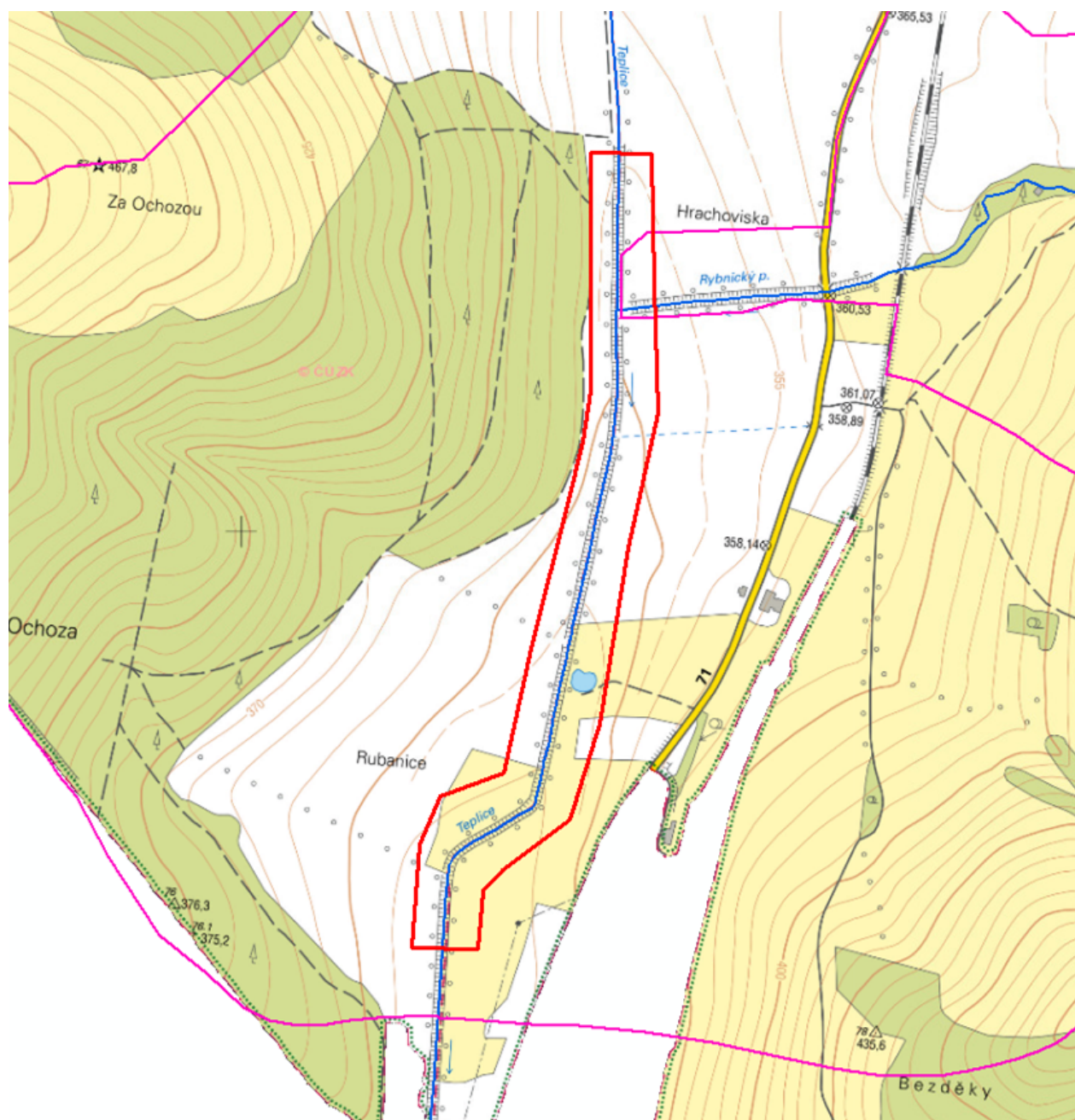
Obrázek 3: Lokalizace navrženého revitalizačního opatření umělé napřímeného koryta Teplice
