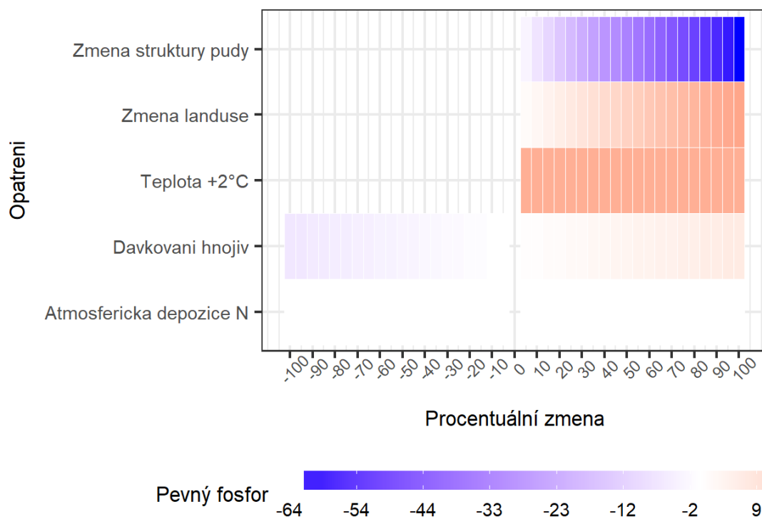
Obrázek 18: Pevný fosfor
