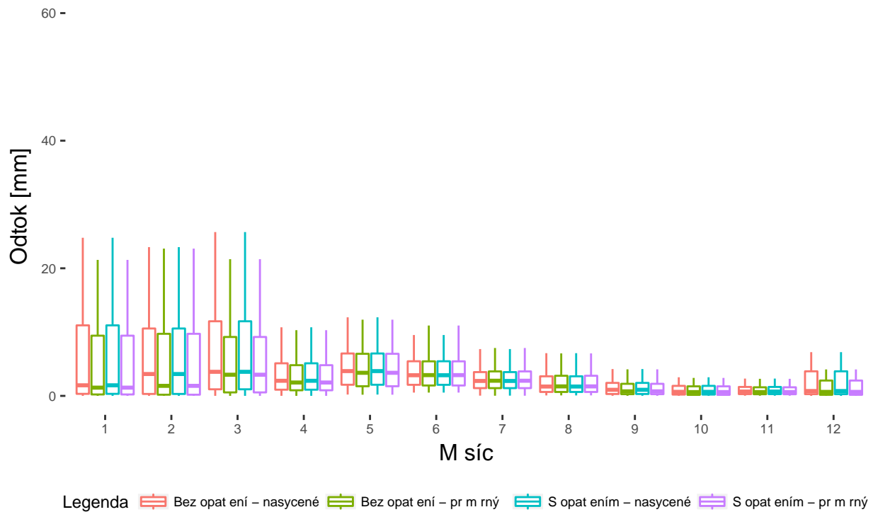
Obrázek 12: Průměrné měsíční odtokové výšky ve formě boxplotů pro jednotlivé varianty hodnocení
