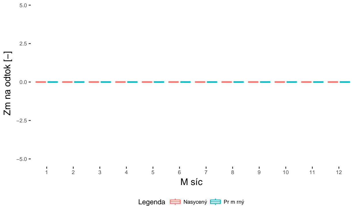
Obrázek 13: Změny měsíčních odtokových výšek ve formě boxplotů (pře opatřením a po realizaci opatření)
